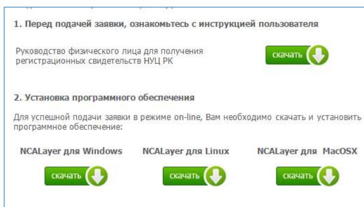
Рисунок 2. Загрузка NCALayer
